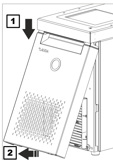
Fig. 78: Enlever le panneau frontal
