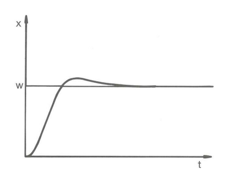
Fig. 62: Paramètre de régulation X_p trop élevé
