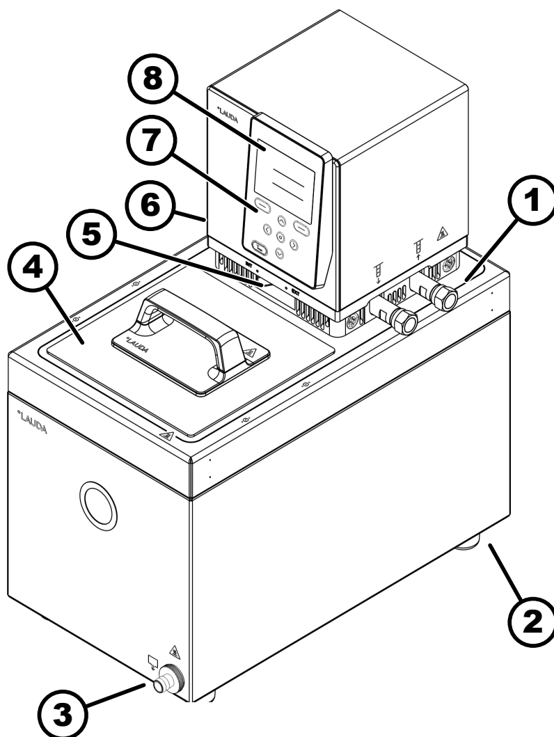
Fig. 12: Thermostat chauffant PRO vue frontale
