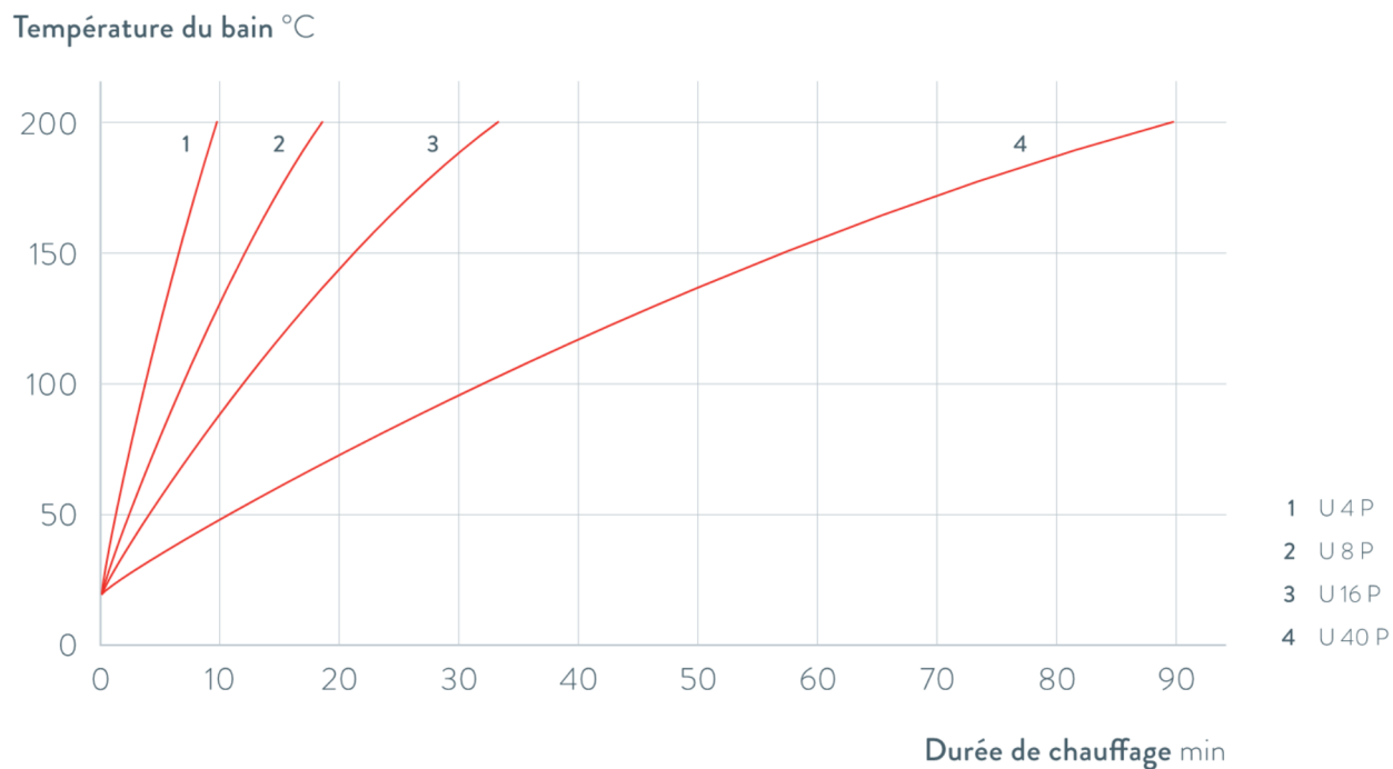
Fig. 81: Courbes de montée en température pour thermostats chauffants Universa PRO
