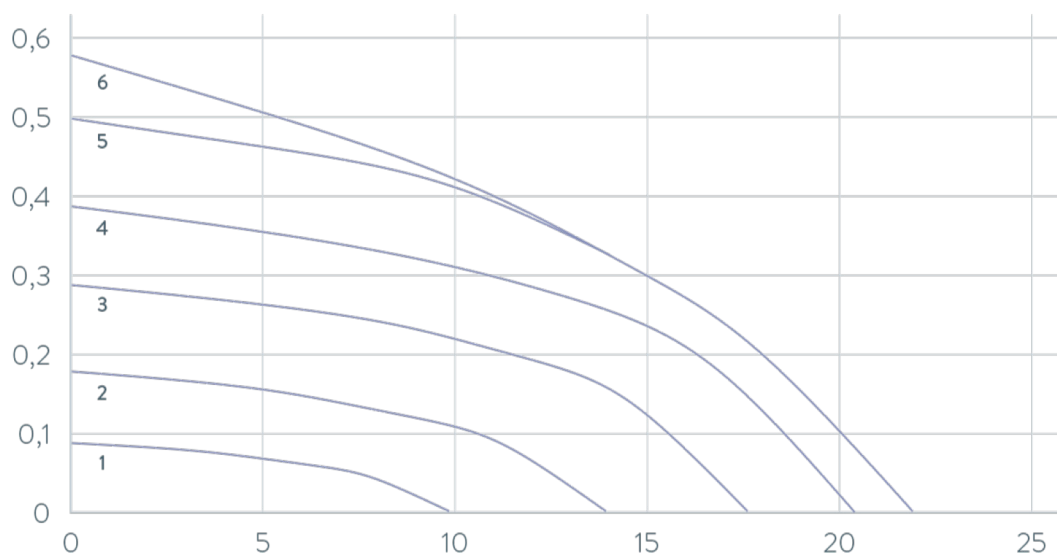
Fig. 85: Caractéristique de la pompe Universa PRO
