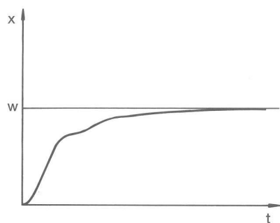
Fig. 65: Paramètres de régulation T_n et T_v trop grands
