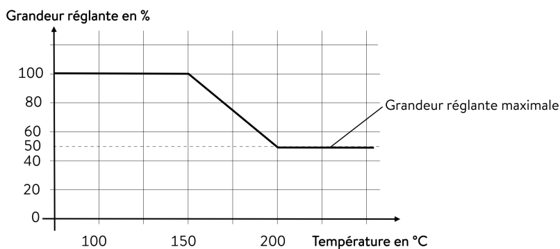
Fig. 68: Limitation dynamique de la puissance de chauffe
