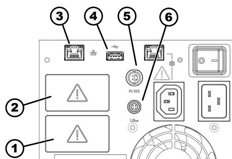
Fig. 14: Interfaces sur l'unité de pompage et de contrôle MAX
