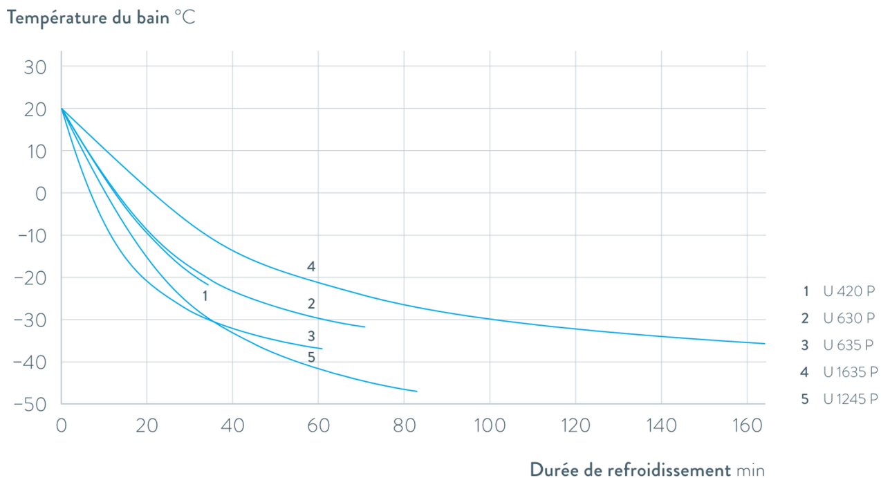
Fig. 83: Courbes de refroidissement pour cryothermostats Universa PRO
