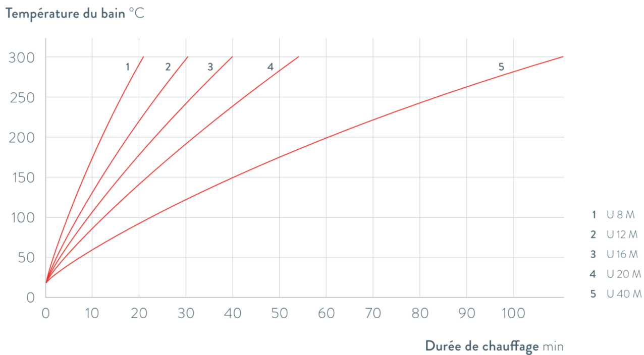
Fig. 82: Courbes de montée en température pour thermostats chauffants Universa MAX
