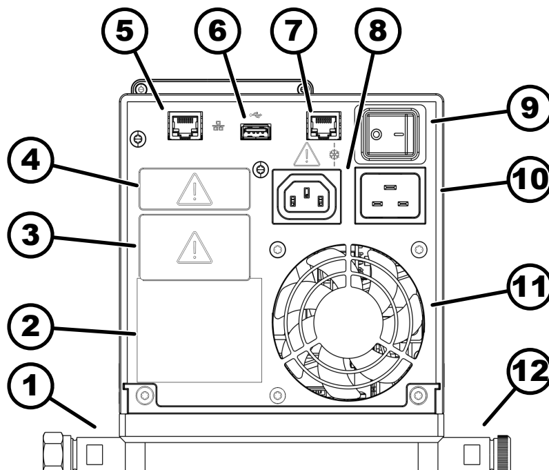
Fig. 10: Unité de pompe et de contrôle Universa PRO, vue arrière
