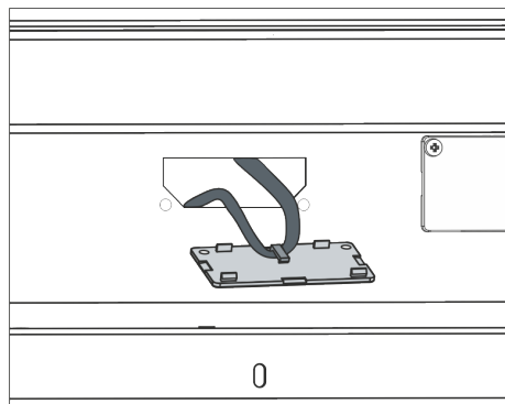
Fig. 27: Détacher le câble-ruban plat LiBus (schéma de principe)
