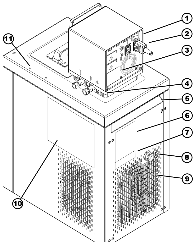
Fig. 8: Cryothermostat MAX, vue arrière
