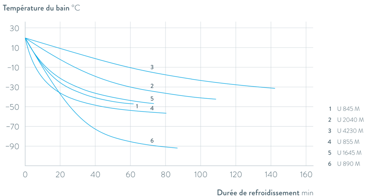
Fig. 84: Courbes de refroidissement pour cryothermostats Universa MAX
