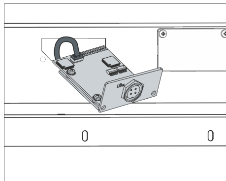
Fig. 28: Raccorder le module d'interface (schéma de principe)
