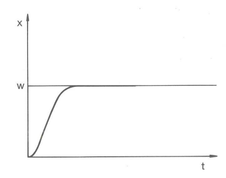
Fig. 61: Réglage optimal
