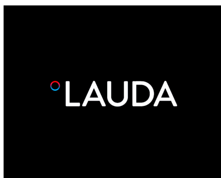
Fig. 34: Écran d'accueil
