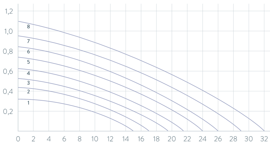
Fig. 86: Caractéristique de la pompe Universa MAX avec pompe de refoulement (pompe Vario) pour une profondeur du bain de 320 mm
