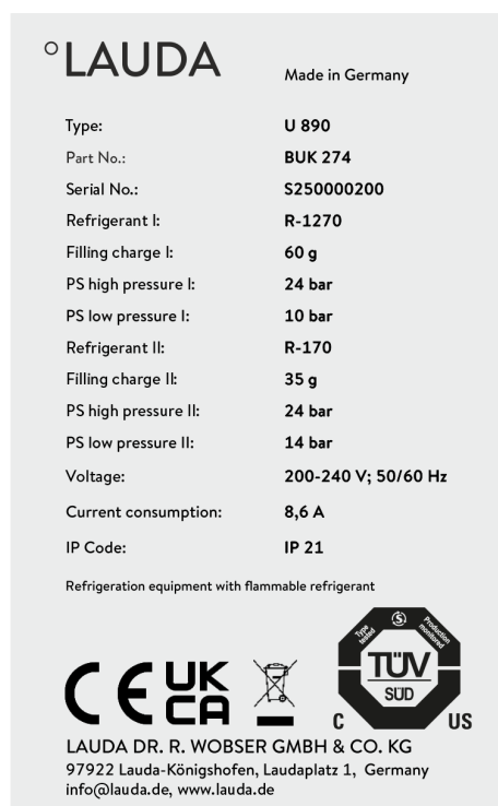
Fig. 18: Plaque signalétique d'un bain de froid
