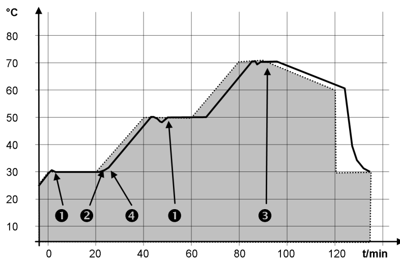
Fig. 74: Déroulement du programme température de consigne et température réelle
