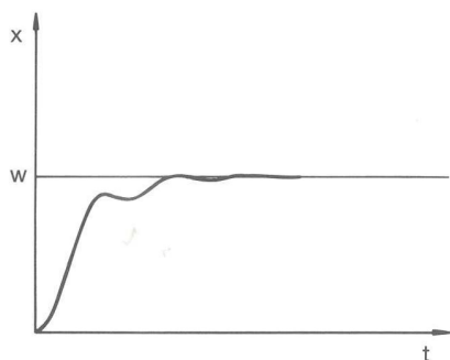
Fig. 63: Paramètre de régulation X_p trop petit
