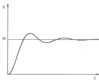
Fig. 64: Paramètres de régulation T_n et T_v trop petits
