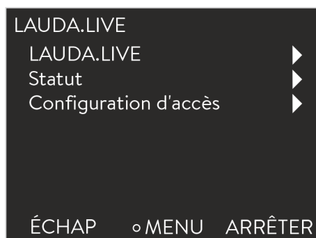
Fig. 21: Menu LAUDA.LIVE
