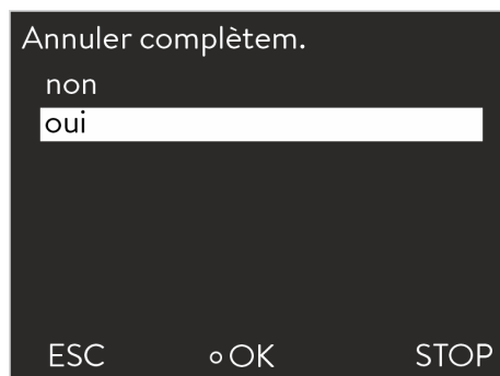
Fig. 54: Paramètres d'usine
