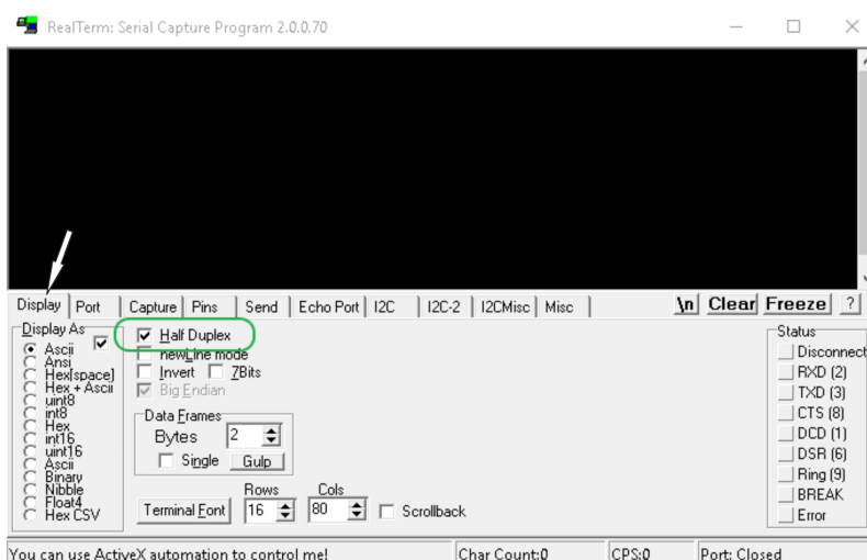
Fig. 49: Programme « RealTerm »
